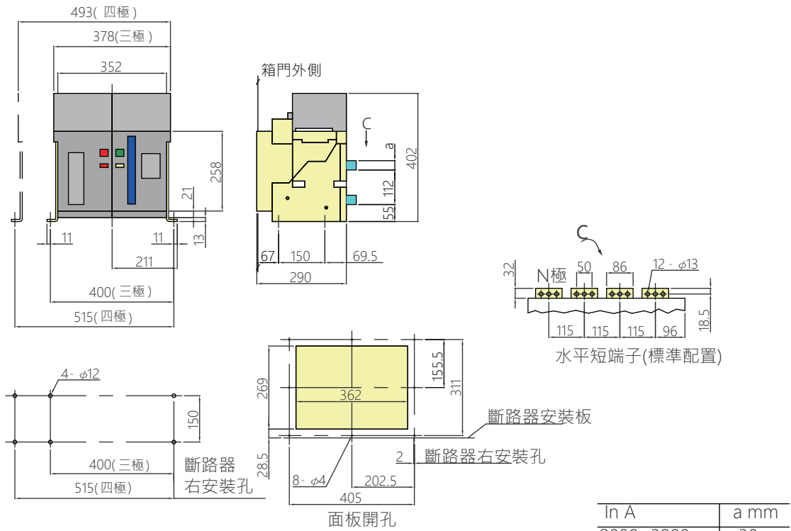
TAB-3200 固定式
