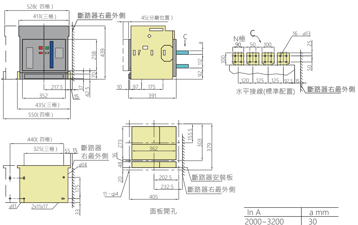
TAB-3200 抽出式
