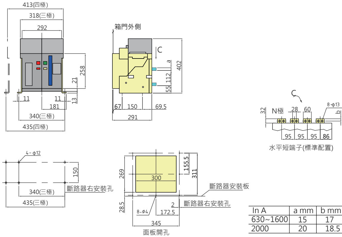
TAB-2000N 固定式
