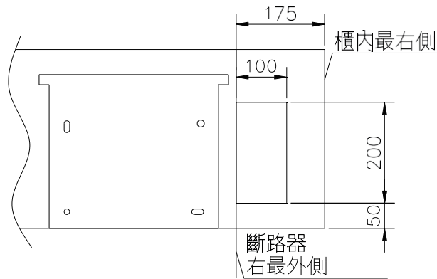
鋼纜連鎖底板開孔尺寸
