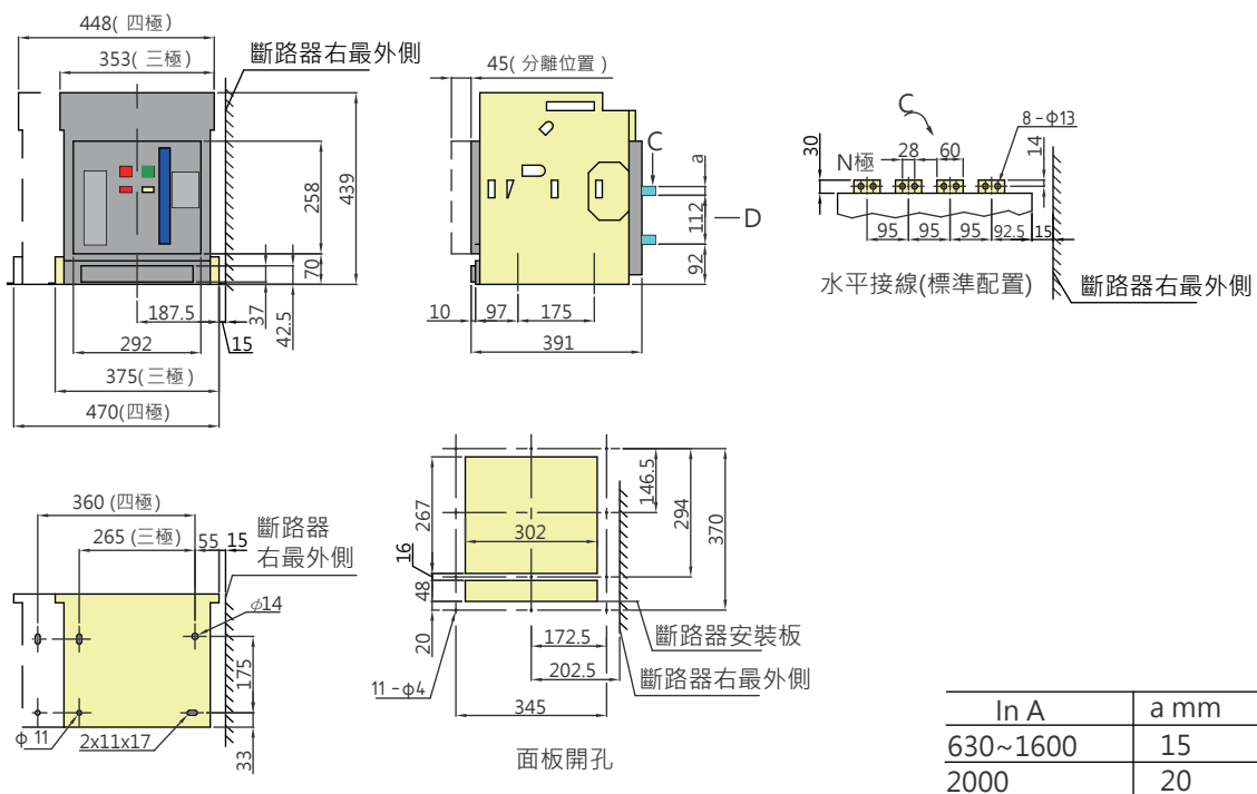
TAB-2000N 抽出式
