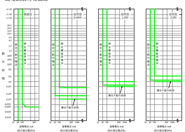
漏電跳脫特性曲線
