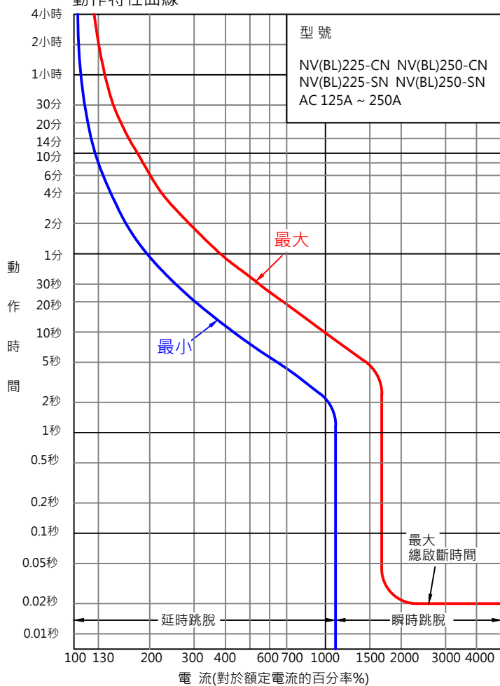
動作特性曲線
