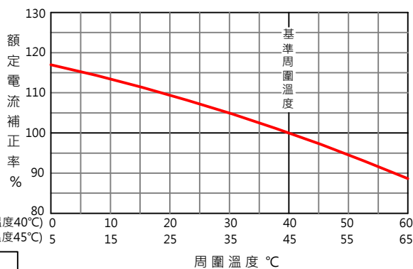
溫度補正曲線
