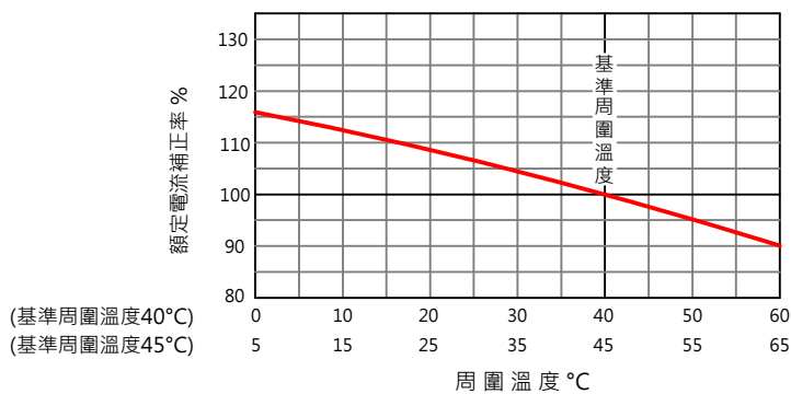
溫度補正曲線
