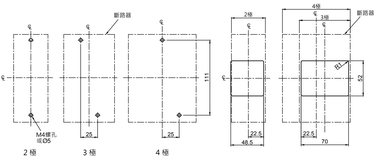
鑽孔圖
