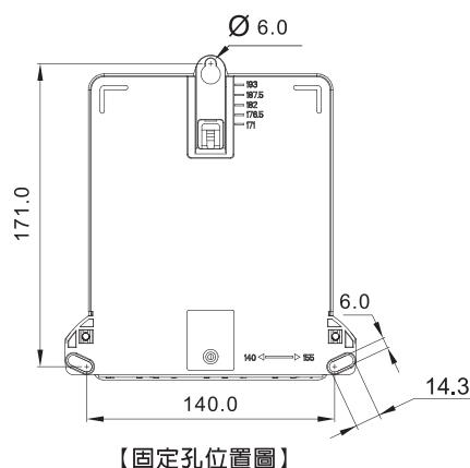
【固定孔位置圖】
