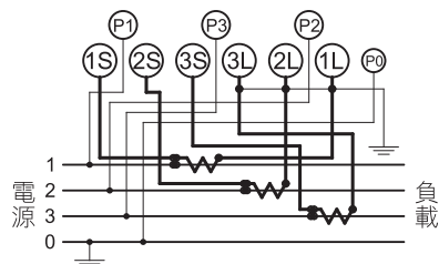
(附變比器用)
