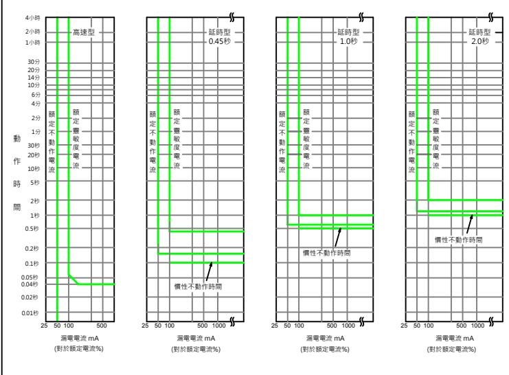
漏電跳脫特性曲線
