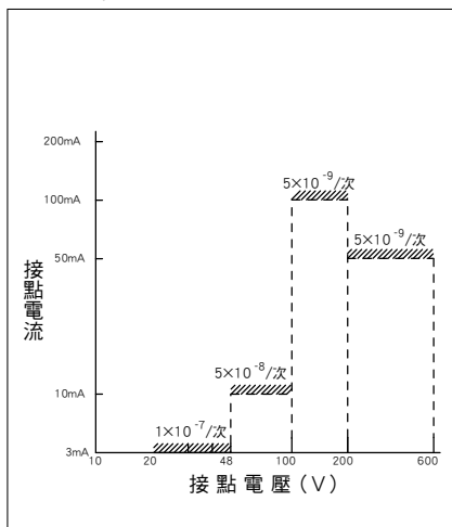
圖4. SR(D)-T5、T9
