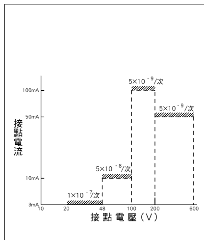
圖2. S(D)-T、UT-Ax11輔助接點
