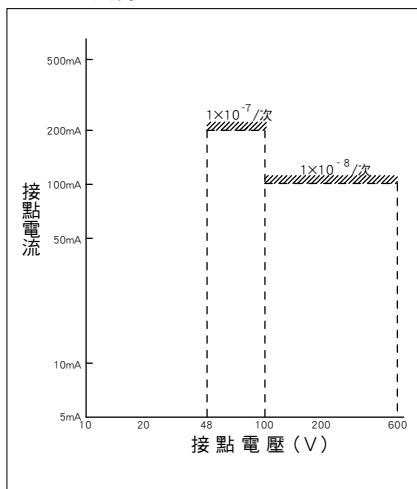
圖1. S(D)-T主接點
