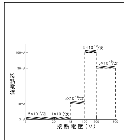
圖3. UT-AX2/4 輔助接點
