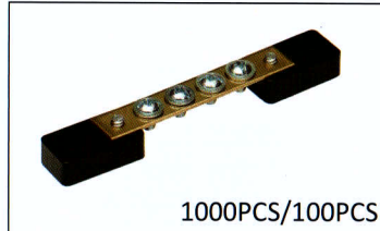
WJ-9204 接地端子板 4P 雙電木 Grounding Terminal Plate
