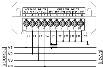
3P4W平衡負載-電壓直入無PT/1CT [設定:3P4W1CT]
