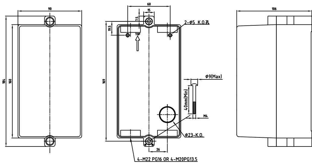
HUP-11,16, HUF-11,16
