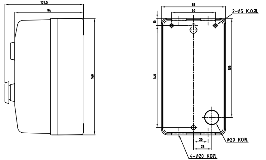
HUEB-11,16
