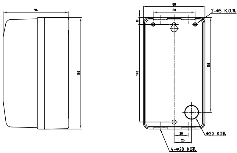
HUE-11,16
