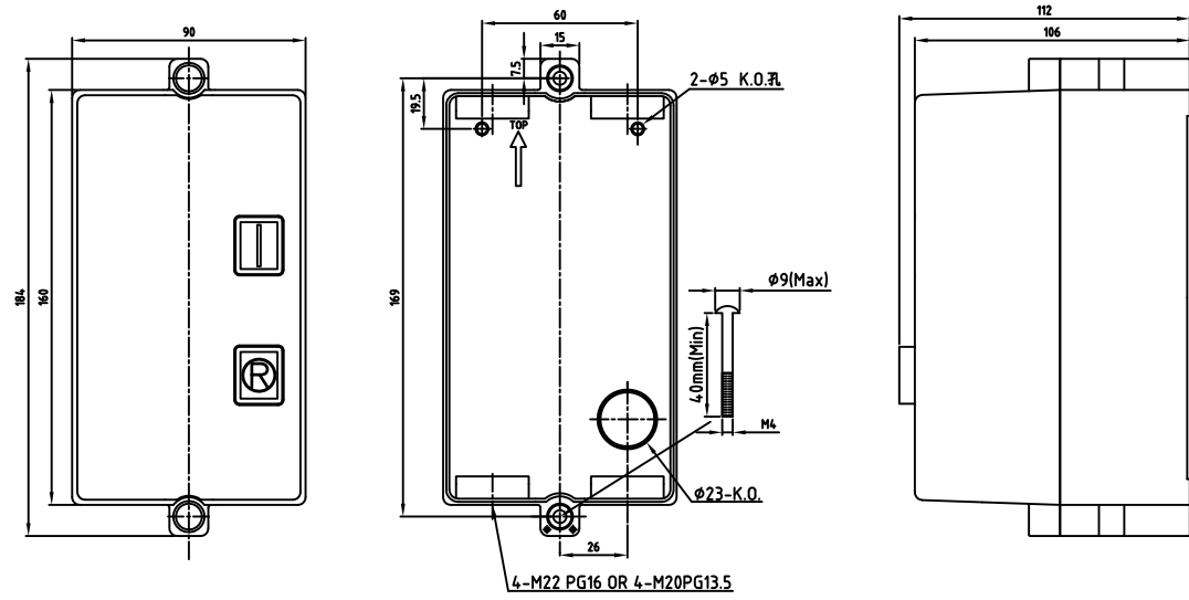
HUPB-11,16, HUFB-11,16
