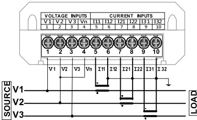
三相三線：無PT/3CT
