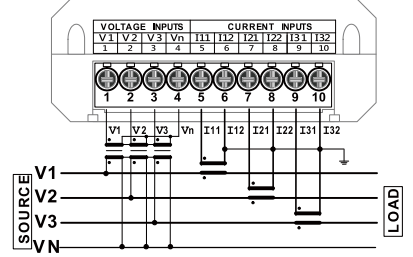
三相四線：無PT/3CT
