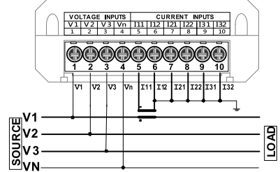
三相四線：無PT/1CT
