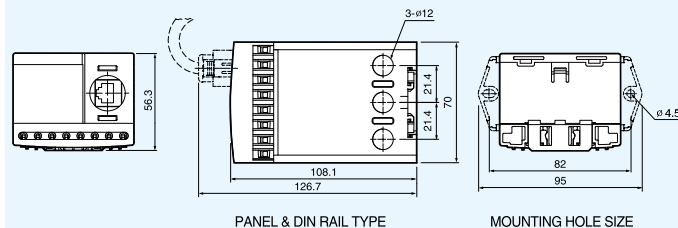
EOCR-FDM2-HZ(過孔式)
