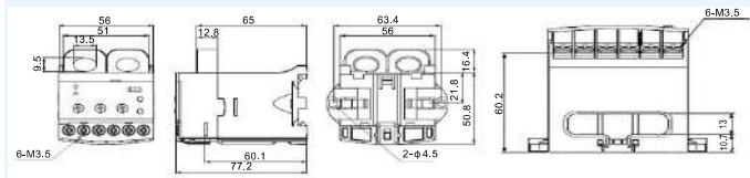
EOCR-SS
