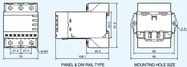
EOCR-3DM2-TZ(端子式)
