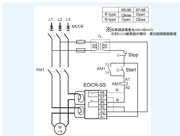
EOCR-SS
