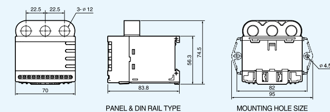
EOCR-i3DM-WZ / i3M420-WZ (穿線式)
