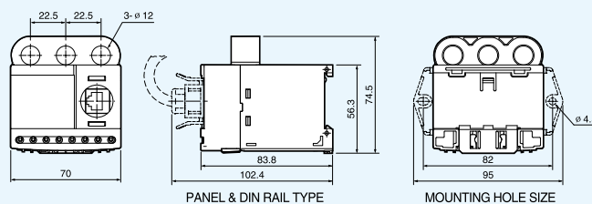
EOCR-FDM2-WZ(穿線式)
