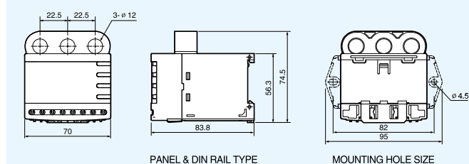
EOCR-3DM2-WZ(穿線式)
