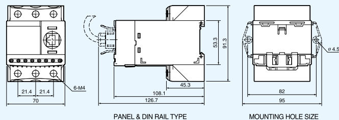
EOCR-FDM2-TZ(端子式)
