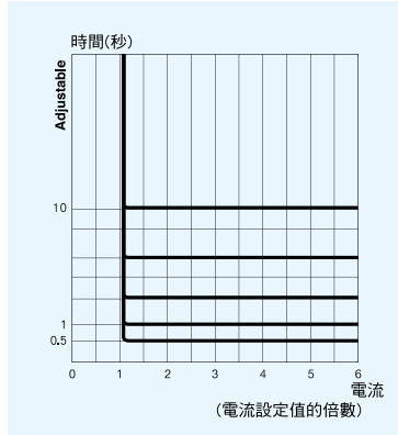
EOCR-SSD的定時限特性
