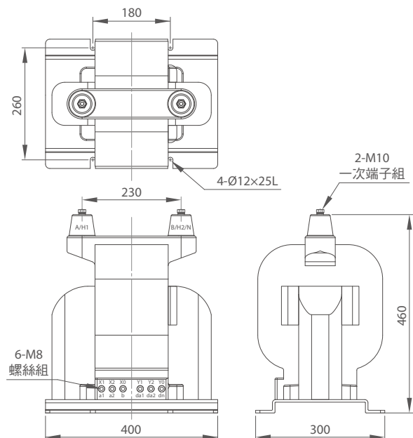
FIG.1 TM-2HF
