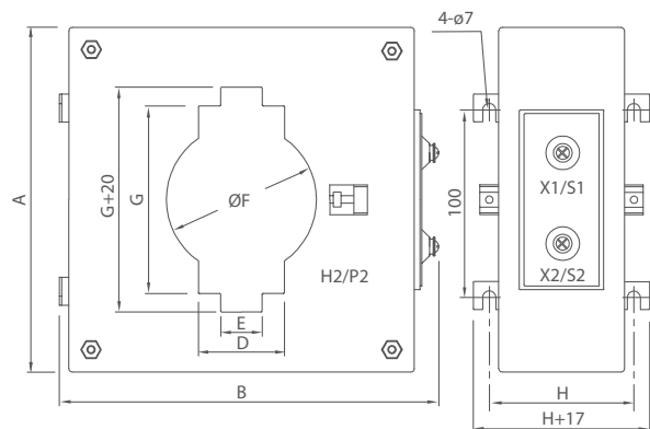
FIG.2 CA-P6, CA-P8
