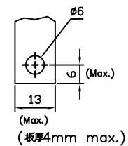
接線端子加工圖
